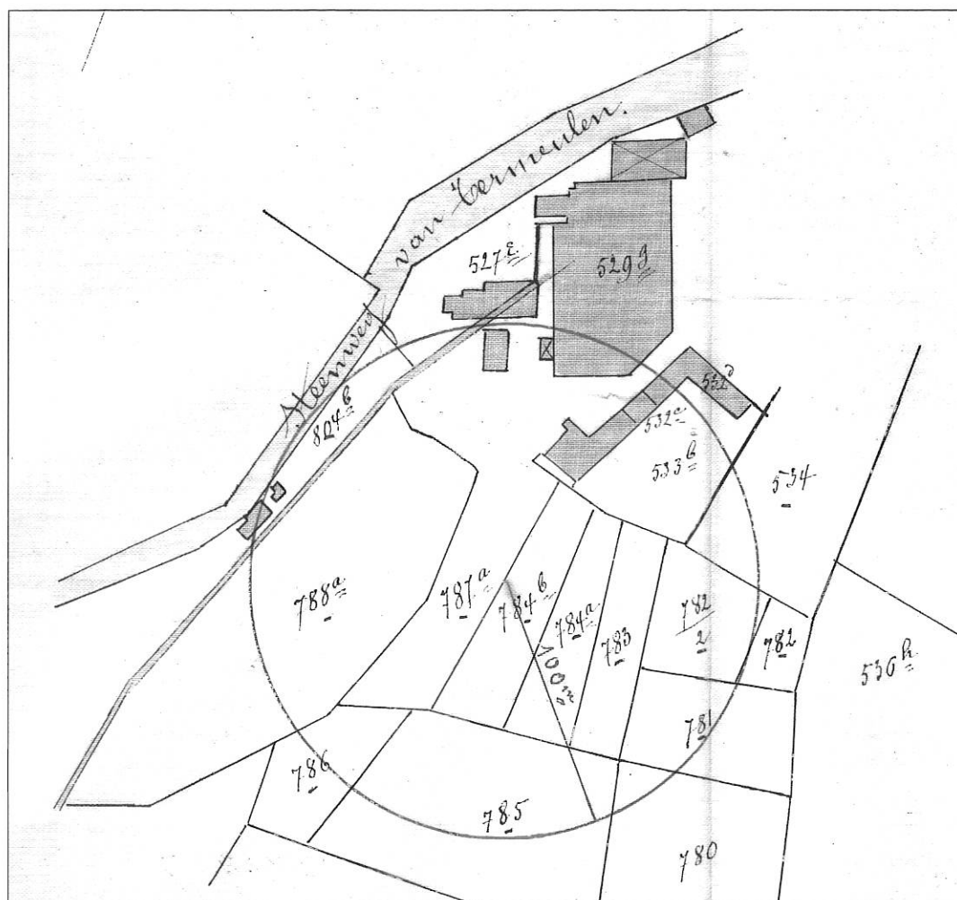
De papierfabriek van de familie de Meurs, voor de vergunning van 1903. Op de kaart ziet men de 100-meterstraal rond de ovens. Deze was nodig om de hinder te berekenen van de omwonenden. Bron: Algemeen Rijksarchief Anderlecht
